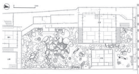
図97 丸井氏庭園配置図 (1/200)
